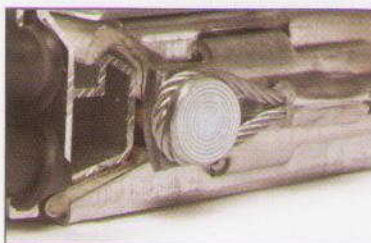
Le câble ne peut être relâché lorsqu'il est sous tension, évitant ainsi tous accidents.
